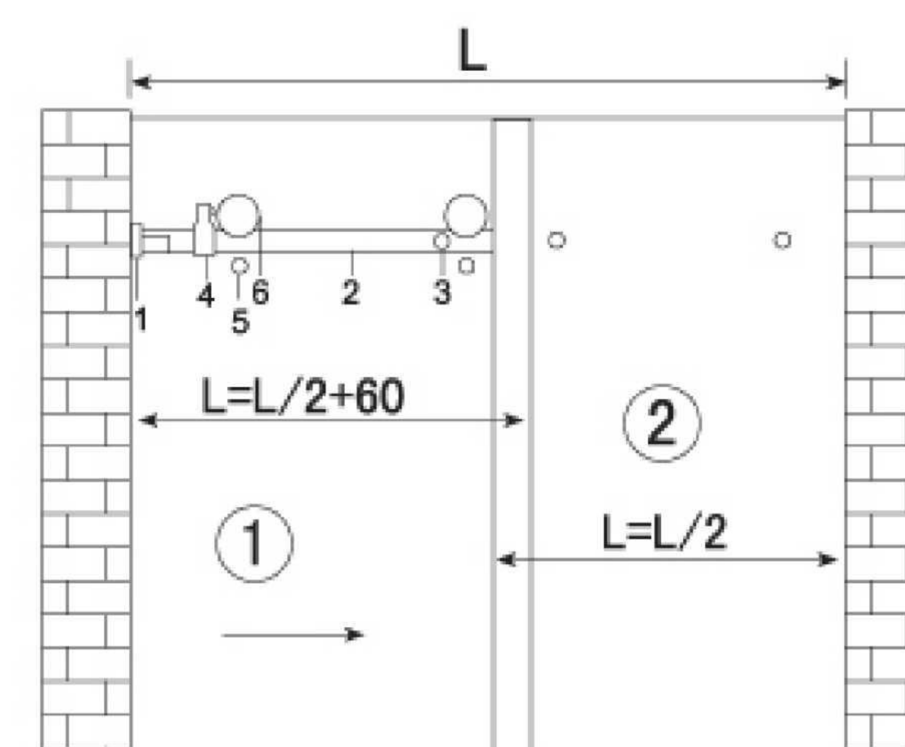
30x15平鵝橢圓管平面安裝圖 30x15 Installation indication of elliptical pipe
