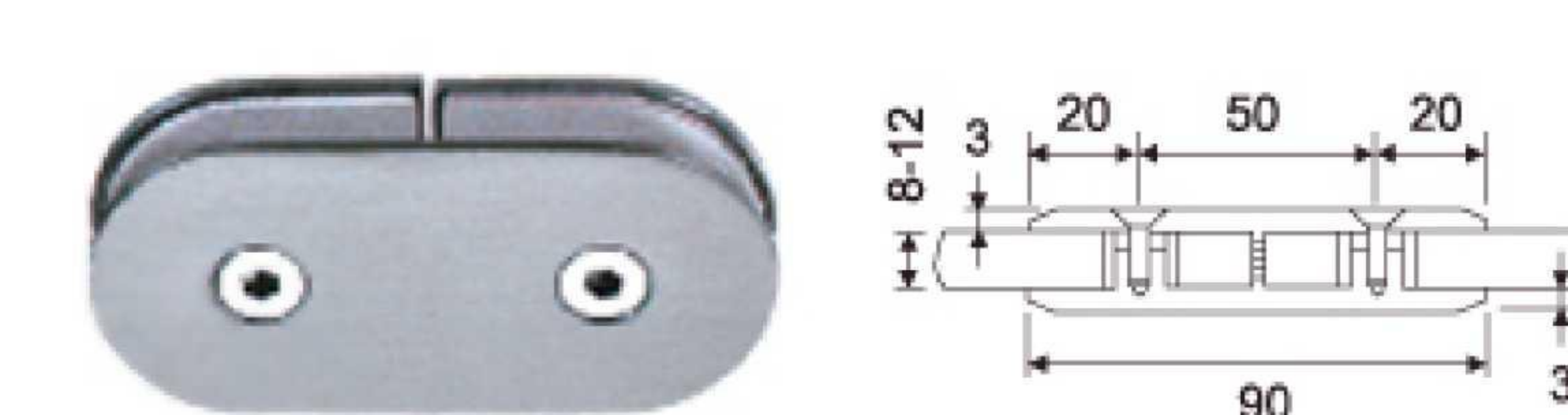
M-508 180° Double Semi-circle
