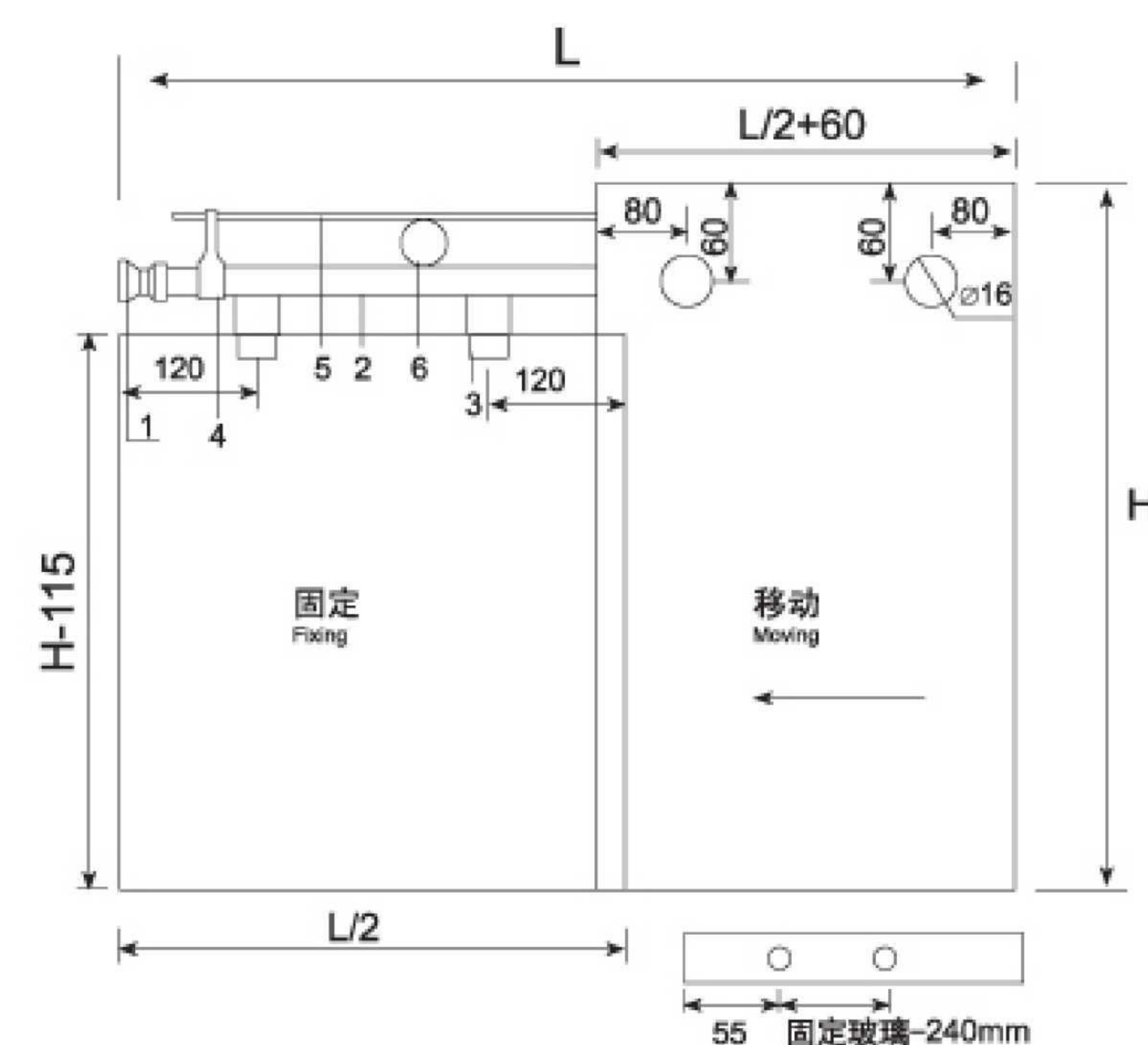
平面安装图 Installation indication
