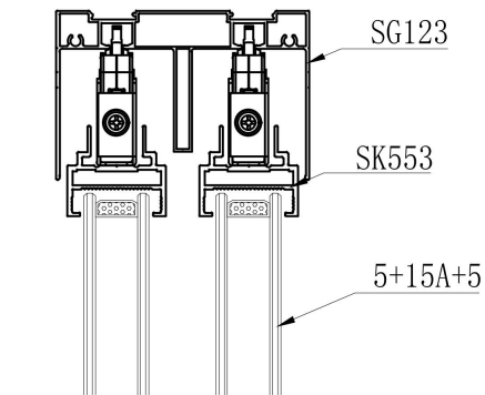
室外: B-B
