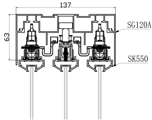
室外: B-B
