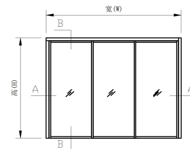
(立面外视图)
