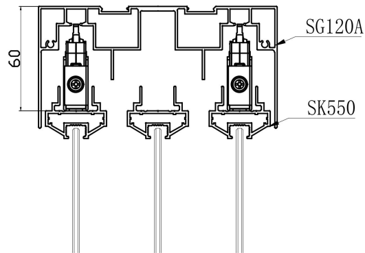
室外: B-B
