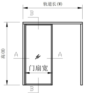
(立面外视图)
