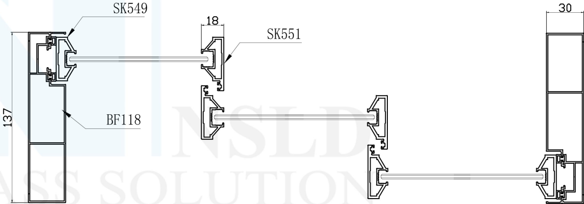
室外: A-A
