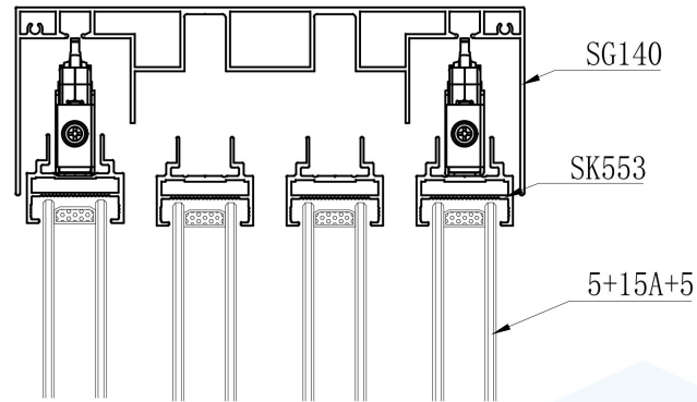
室外: B-B
