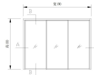
(立面外视图)
