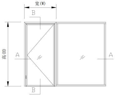
(立面外视图)
