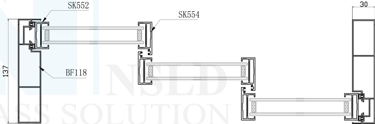
室外: A-A
