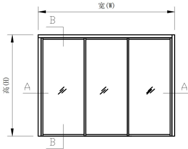
(立面外视图)
