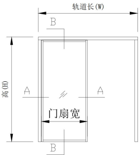
(立面外视图)
