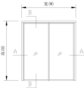
(立面外视图)
