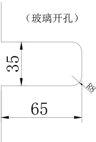
(立面外视图)
