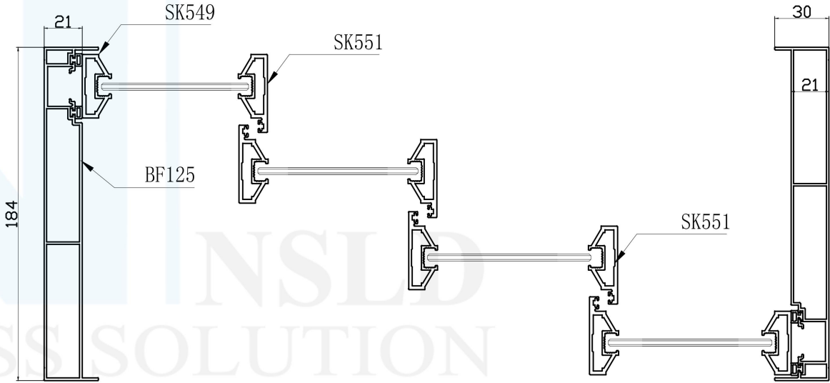
室外: A-A
