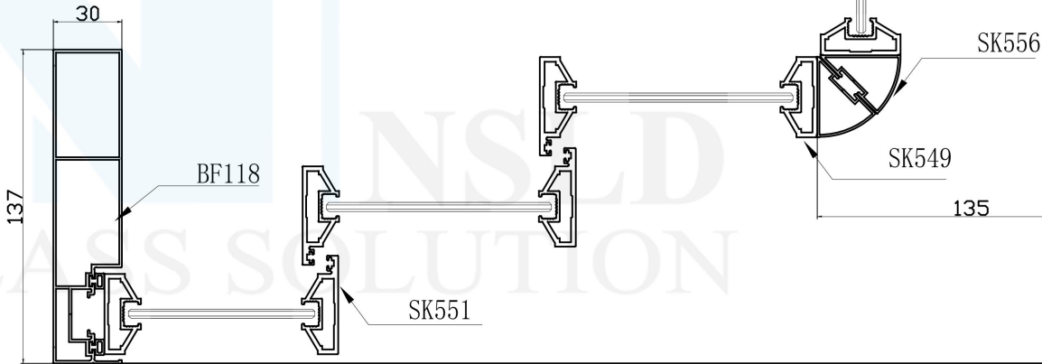
室外: A-A
