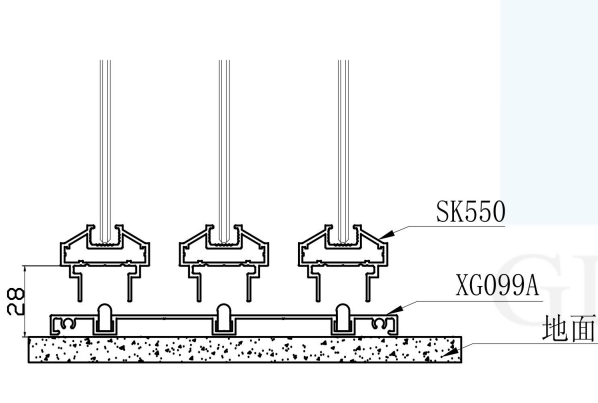
室外: B-B
