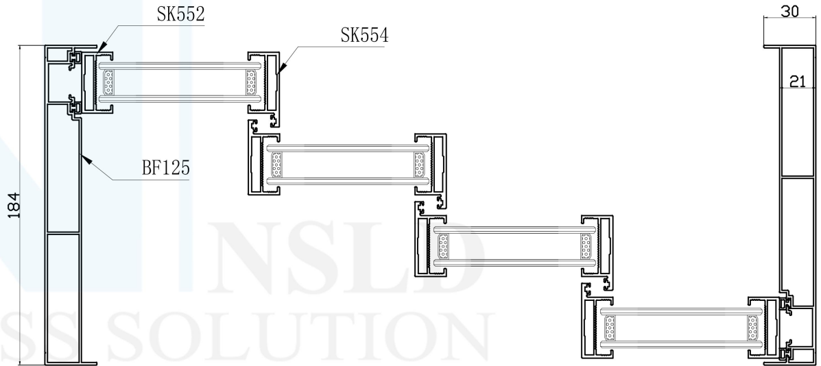
室外: A-A
