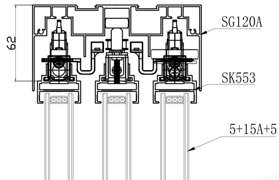
室外: B-B
