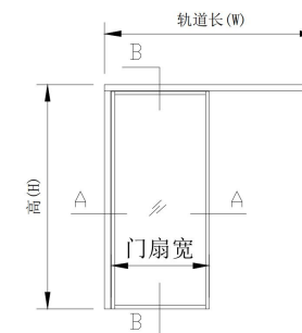
(立面外视图)
