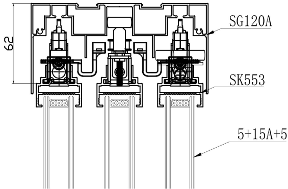
室外: B-B
