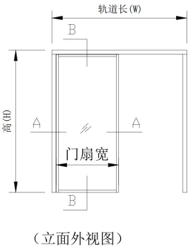
(立面外视图)
