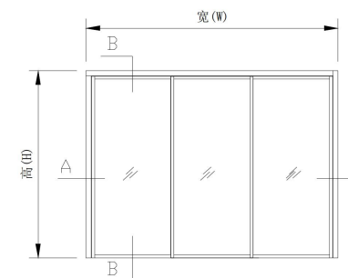
(立面外视图)
