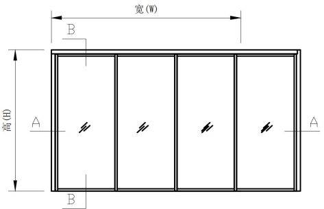
(立面外视图)
