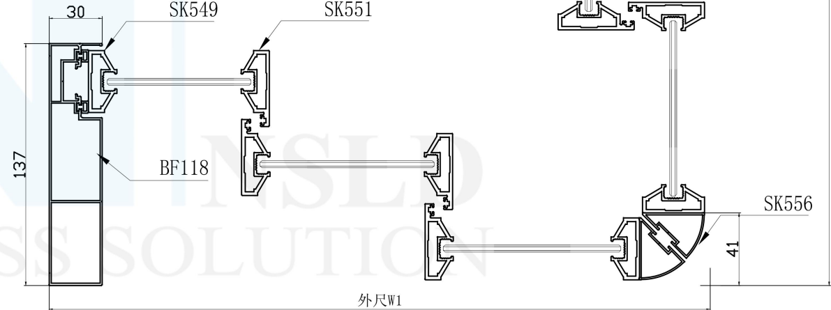
室外: A-A
