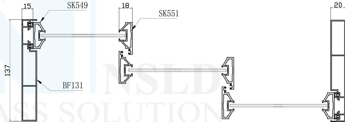
室外: A-A
