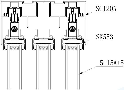
室外: B-B
