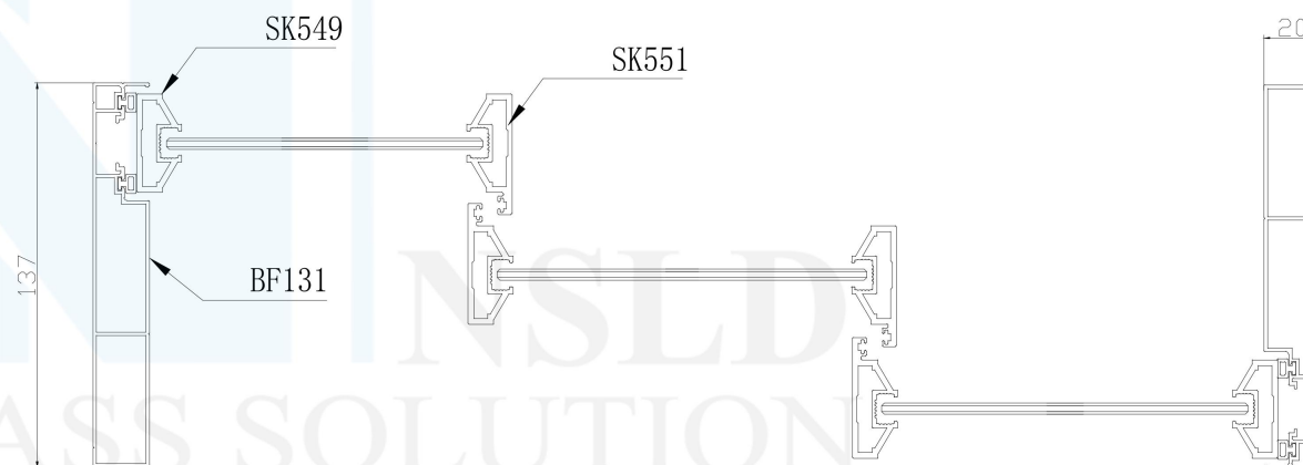
室外: A-A
