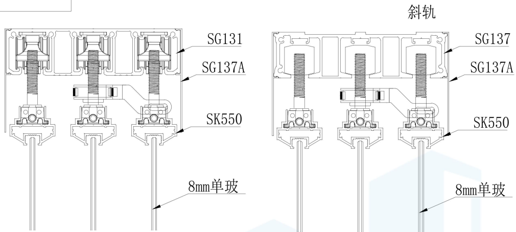
室外: B-B
