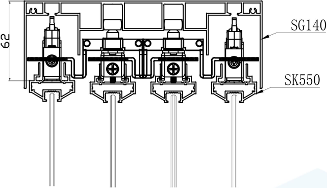
室外: B-B
